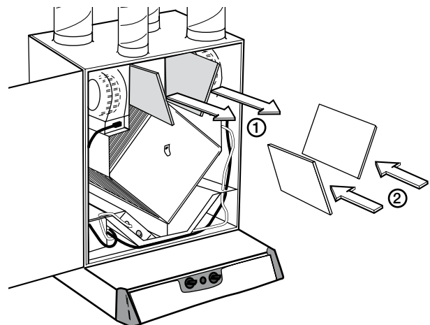
Figur 13. Filtrens placering i aggregatet. (Observera att filtren kan vara av annan typ än de som visas i illustrationen ovan).
