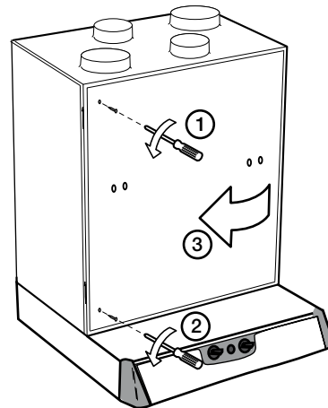
Figur 12. Öppning av aggregatluckan.
